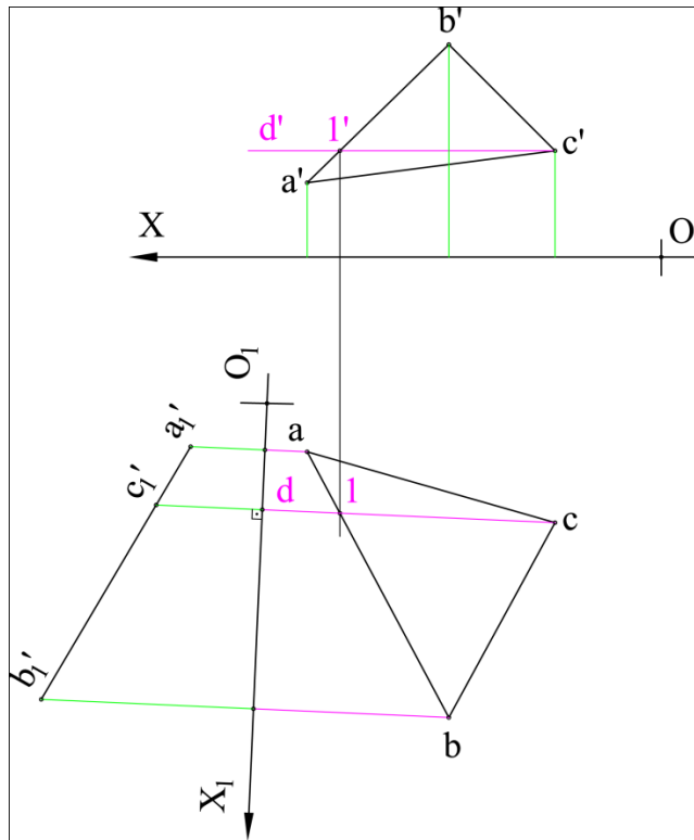
3. Proiecția pe noul plan a plăcii triunghiulare în funcție de cotele punctelor
