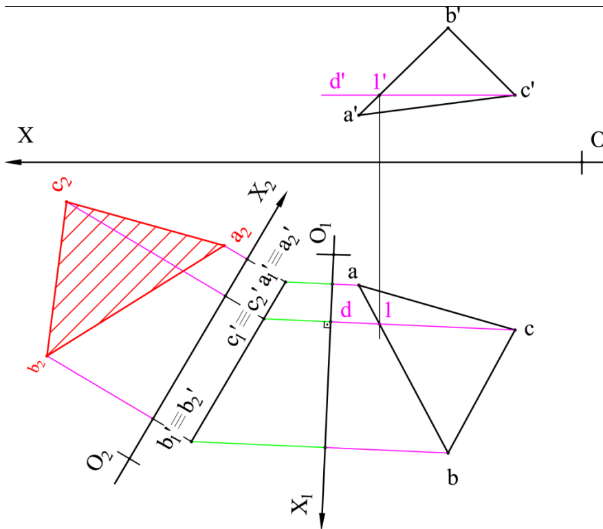
5. Adevărata mărime a triunghiului ABC prin dubla schimbare a planelor de proiecție
